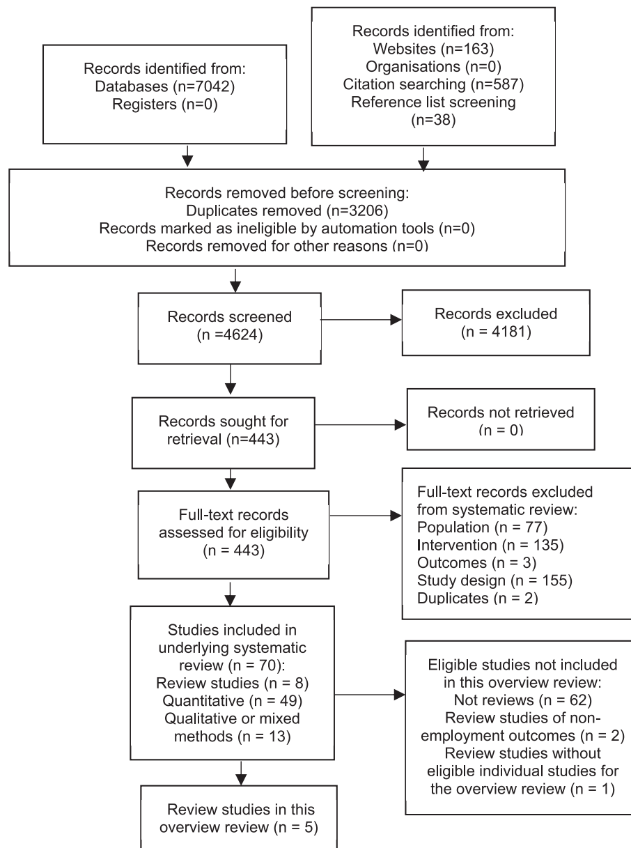
Fig. 1. PRISMA diagram.
